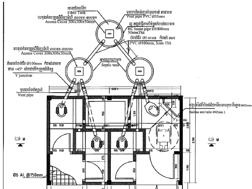
Plan des connexions des toilettes avec les fosses septiques et le réservoir de filtration avant évacuation dans la nature
